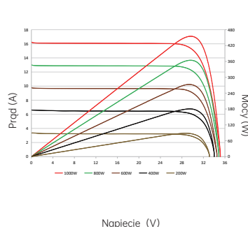
Charakterystyka prądowo - napięciowa (445W)
